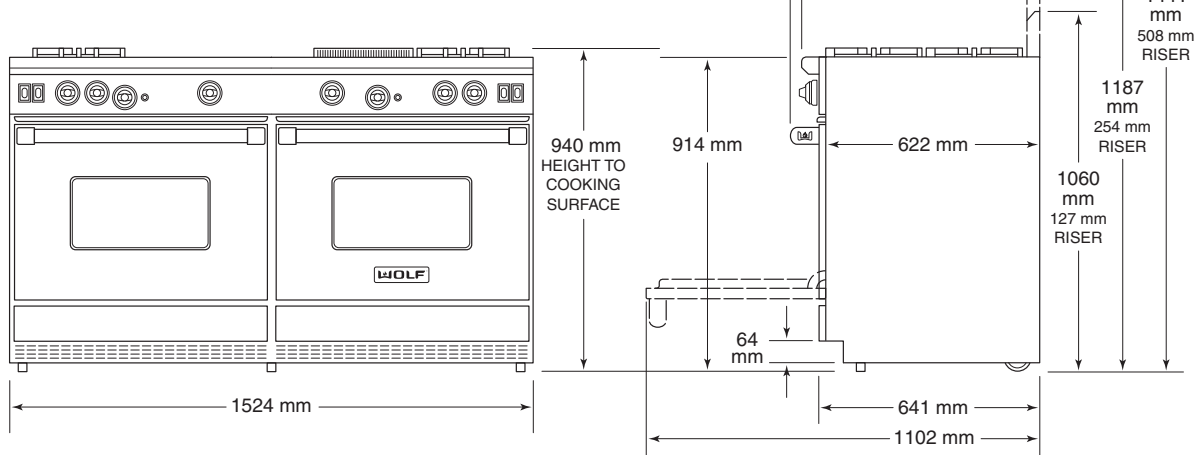
1527 mm RANGE
