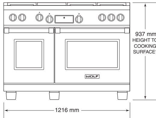
1219 mm RANGE
